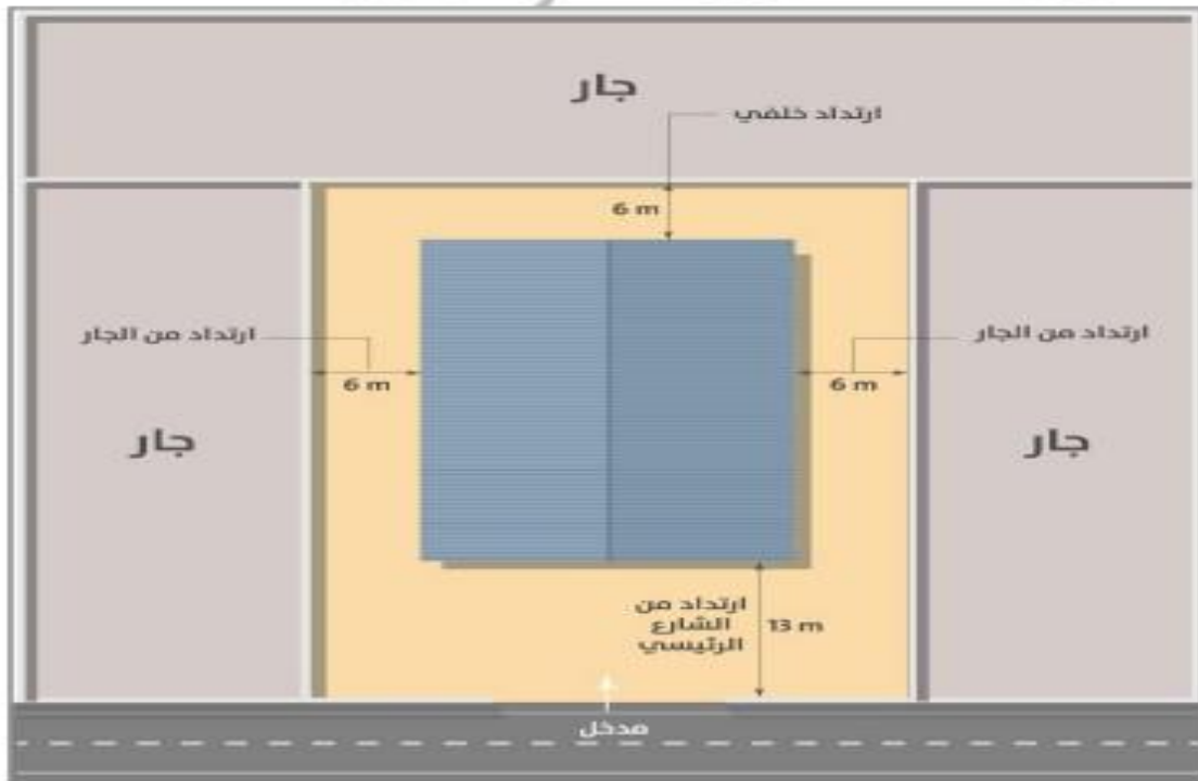
مثال (ب) يوضح الارتدادات في المواقع المعتمدة كمخططات للمصانع
