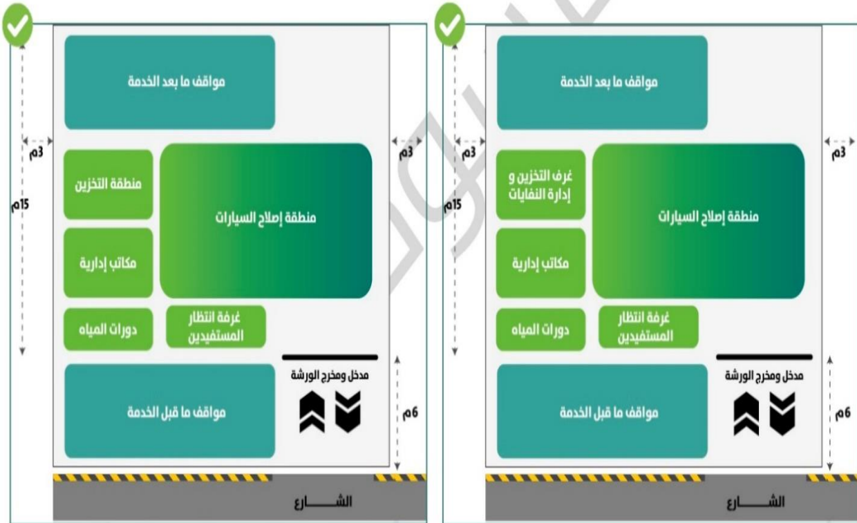
شكل توضيحي (1): نموذج استرشادي لتصميم ورشة إصلاح مركبات
