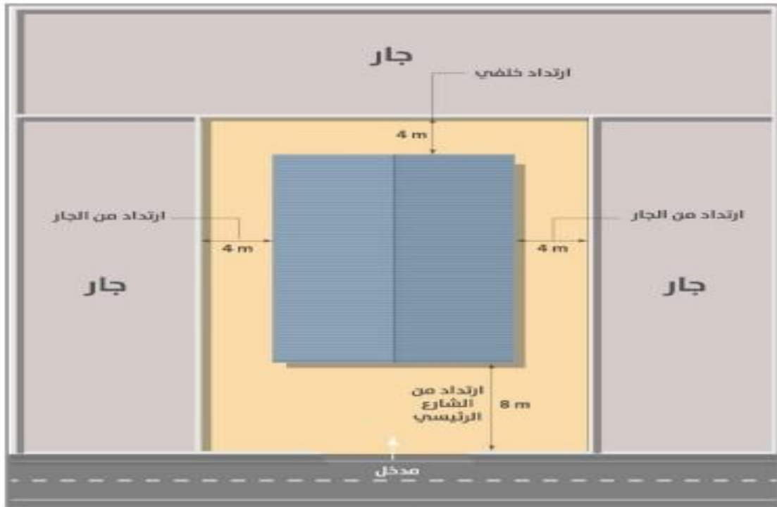
مثال (أ) يوضح الارتدادات لموقع مستقل ومناطق الخدمات المساندة
