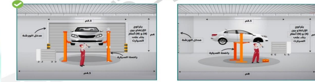
شكل توضيحي (3): رسم توضيحي جانبي وعلوي لقياسات قسم صيانة السيارات
